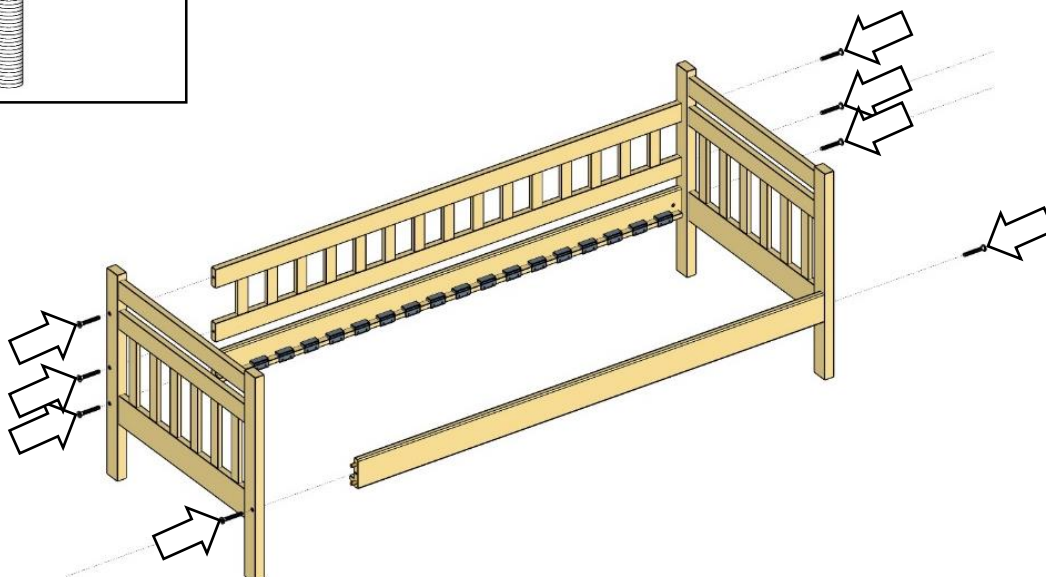
M6x80
