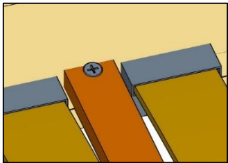
Шуруп 3,5x25
