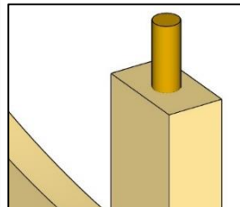
Шкант 12x70
