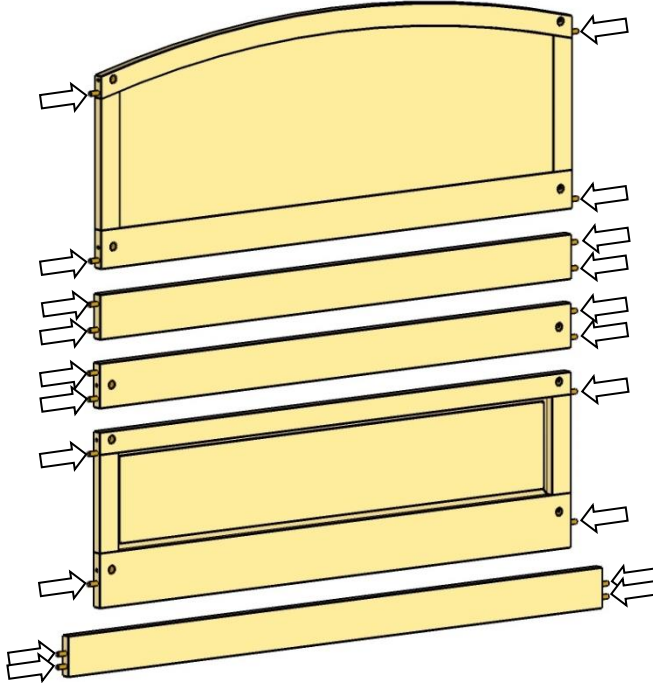
Шкант 10x50
