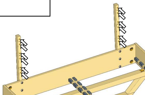
Шканти 8х35
